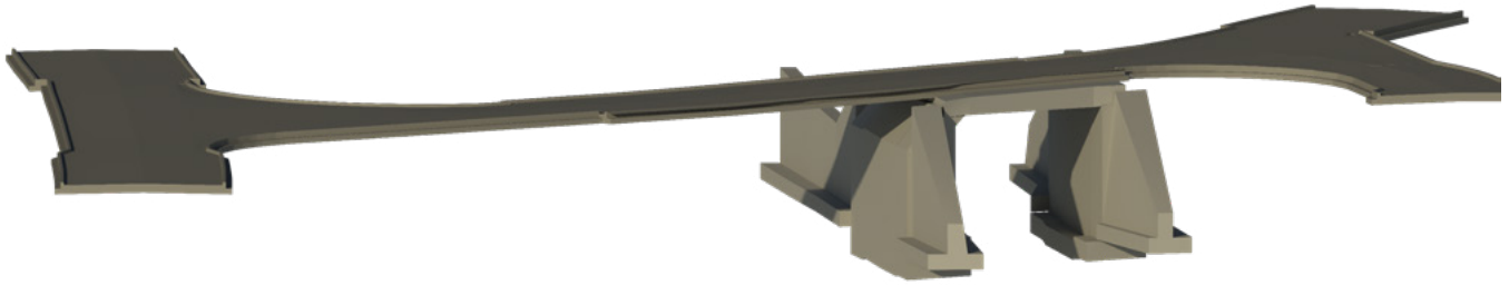
Abbildung 22: BIM-Modell des Brückenbauwerks und des Straßenabschnitts des Pilotprojekts „Brücke Bielefelder Straße“ 120
