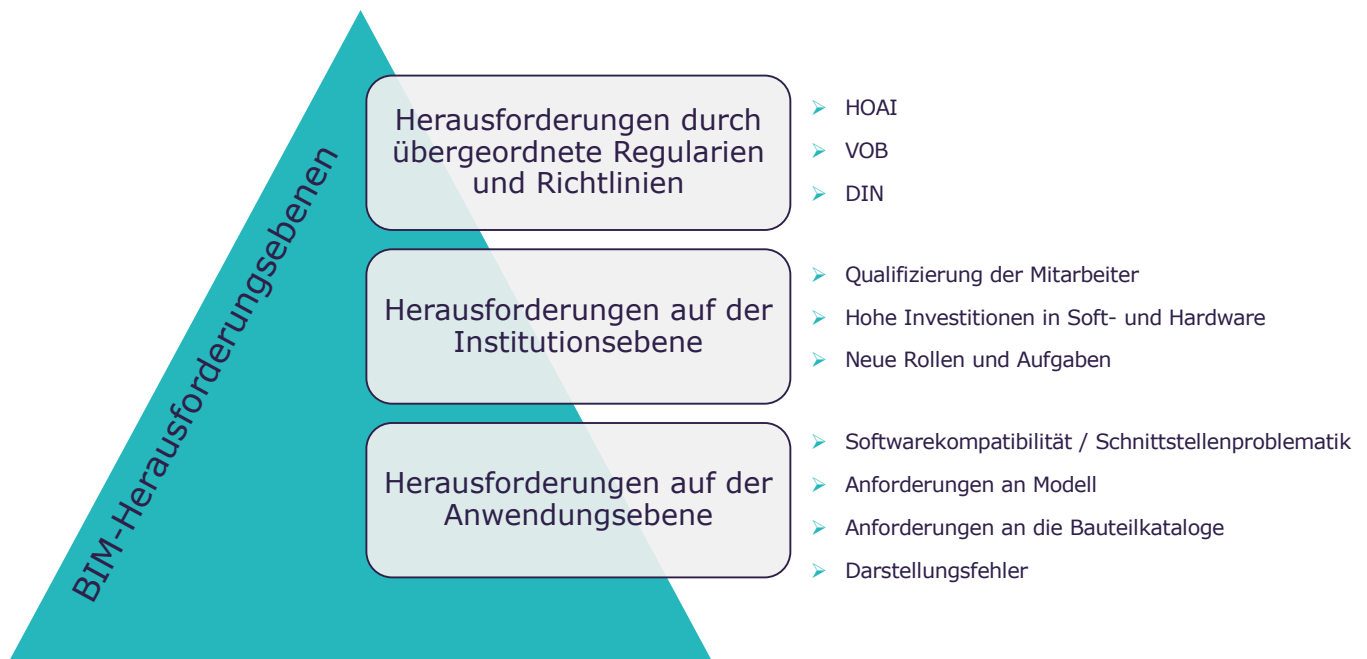
Abbildung 14: Allgemeine Herausforderungsebenen 99
